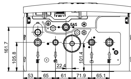
Onderaanzicht van modellen D2TND012A4AB, D2TND018A4AB en D2TND024A4AB
