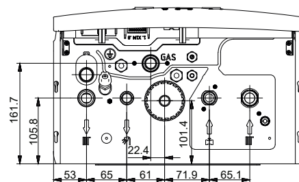
Onderaanzicht van model D2CND024A4AB
