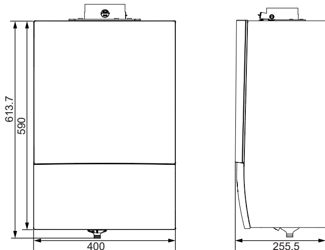
Onderaanzicht van model D2CND024A1AB
