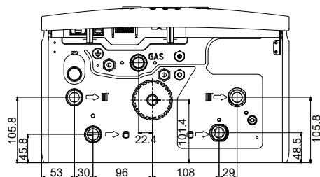
Onderaanzicht van modellen D2TND012A4AB, D2TND018A4AB en D2TND024A4AB
