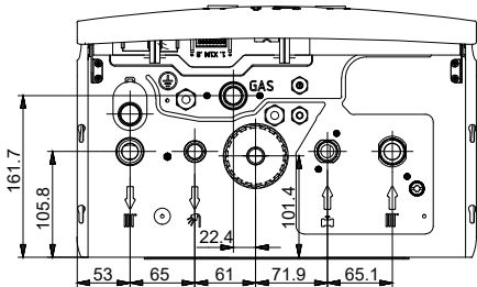
Vista inferior del modelo D2CND024A4AB
