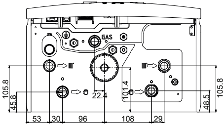
Vista inferior de los modelos D2TND012A4AB, D2TND018A4AB y D2TND024A4AB
