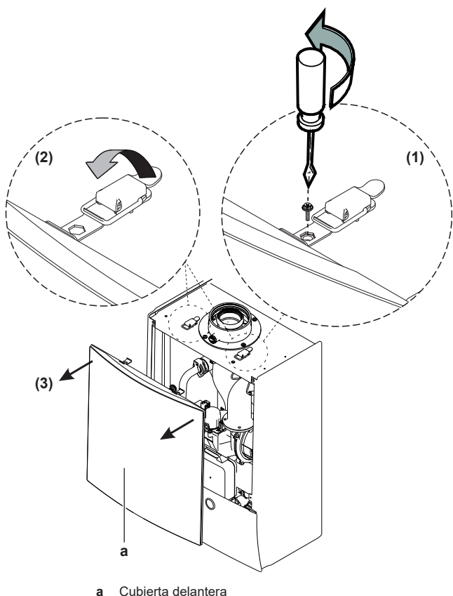
a Cubierta delantera
