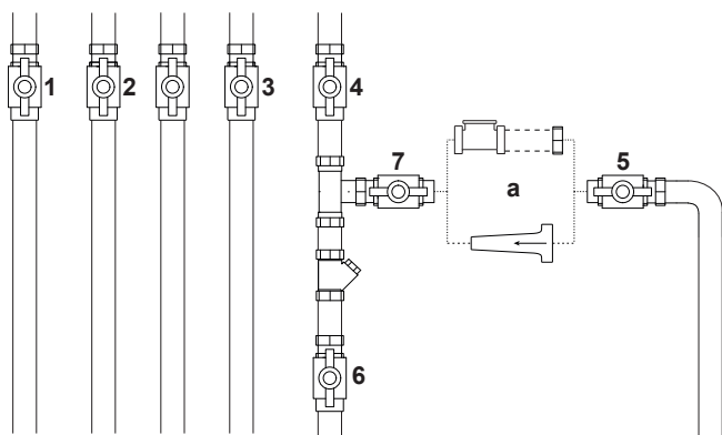
a Използвайте разединител или двоен възвратен вентил съгласно местните разпоредби
