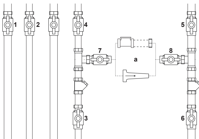
a Използвайте разединител или двоен възвратен вентил съгласно местните разпоредби
