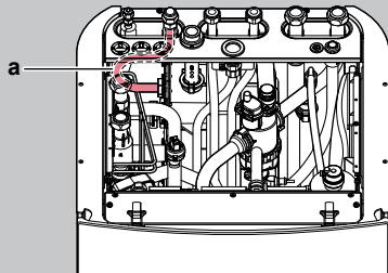
a Soğutucu akışkan gaz borusu
