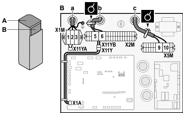
a Соединительный кабель (=основное электропитание) b Источник электропитания по обычному тарифу c Контакт подачи электропитания с предпочтительным энергосбережением
