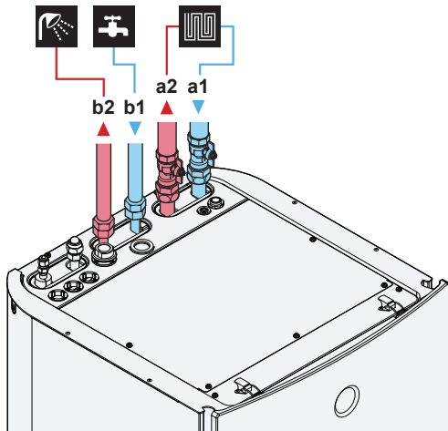
a1 Térfűtés/hűtés – Víz BEMENETE (csavarkötés, 1") a2 Térfűtés/hűtés – Víz KIMENETE (csavarkötés, 1")
