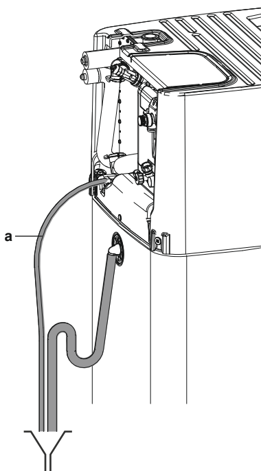
a Шланг дренажного поддона
