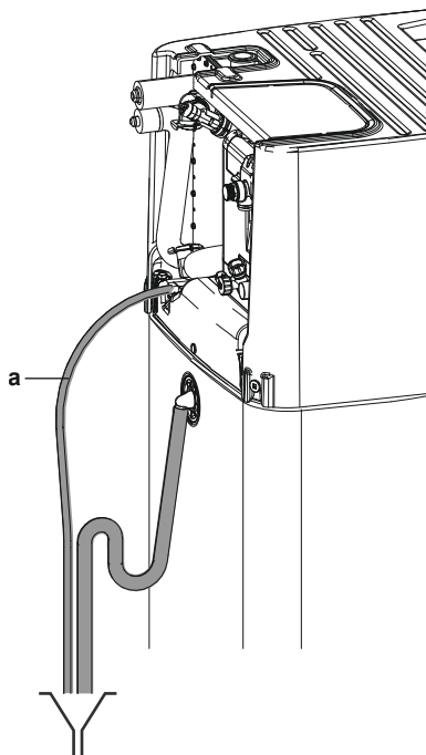
a Furtunul tăvii de evacuare
