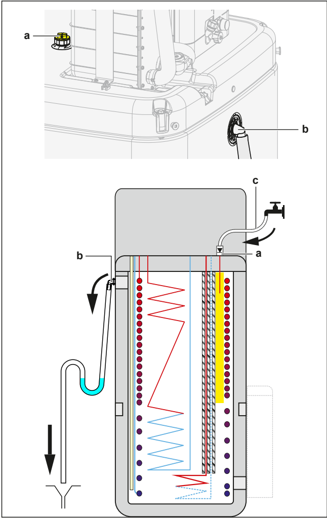
a Tilbakerenningskobling b Overflommingskobling c Slange med tilbakeslagsventil (1/2")
