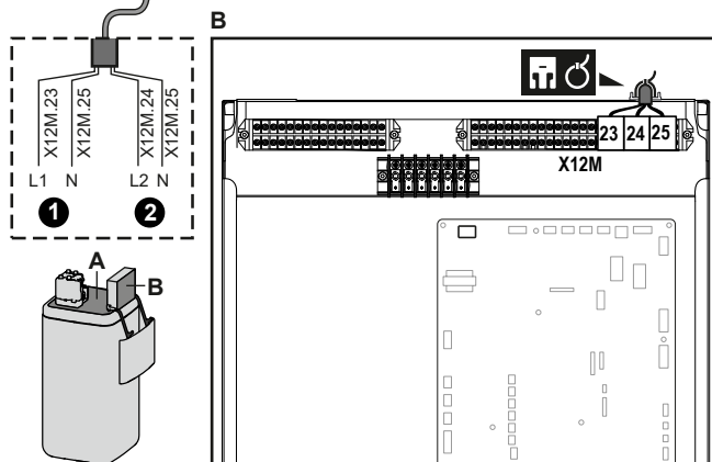
6 Kiinnitä kaapeli nippusiteillä nippusiteiden kiinnikkeisiin. Yleistä tietoa varten katso "6.3.1 Sähköjohtojen liittäminen sisäyksikköön" [21].
