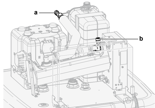
a, b Ръчен вентил на отворите за излизане на въздух
