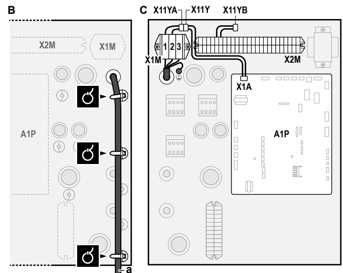
a Соединительный кабель (=основное электропитание)
