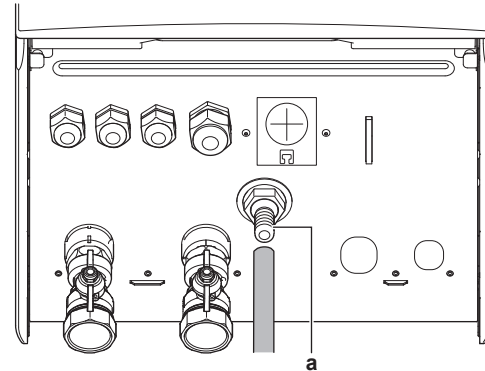
а Конектор за дренажната тава
