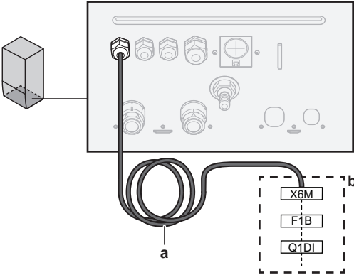
a Фабрично монтиран кабел, свързан към контактора за резервния нагревател, вътре в превключвателната кутия (K5M) b Окабеляване на място (вижте таблицата по-долу)
