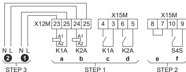
STEP 1 Montering av Smart Grid-reläsetsen
