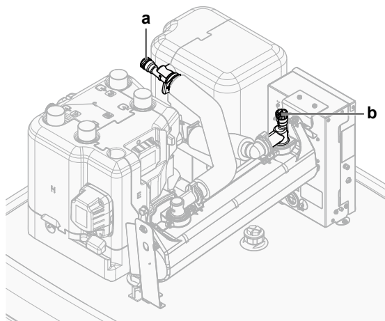
a, b Ręczny zawór odpowietrzający
