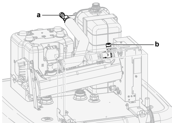
a, b Válvula de purga de ar manual
