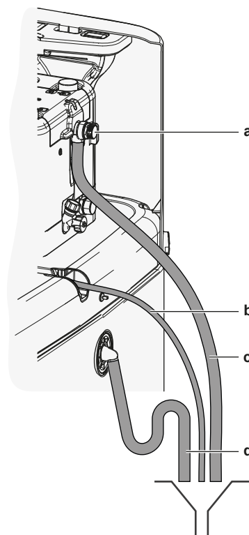
a Slėgio mažinimo vožtuvas b Išleidimo padėklo žarna (pristatoma kaip priedas) c Išleidimo žarnos slėgio mažinimo vožtuvas (išsigijamas atskirai) d Išleidimo žarnos bakas (išsigijamas atskirai)
