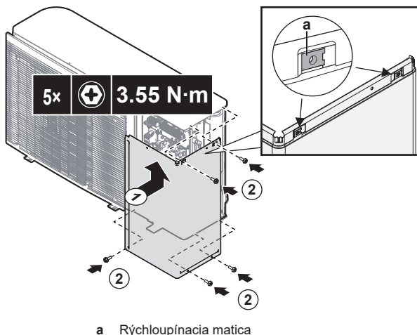
a Rýchlopínacia matica
