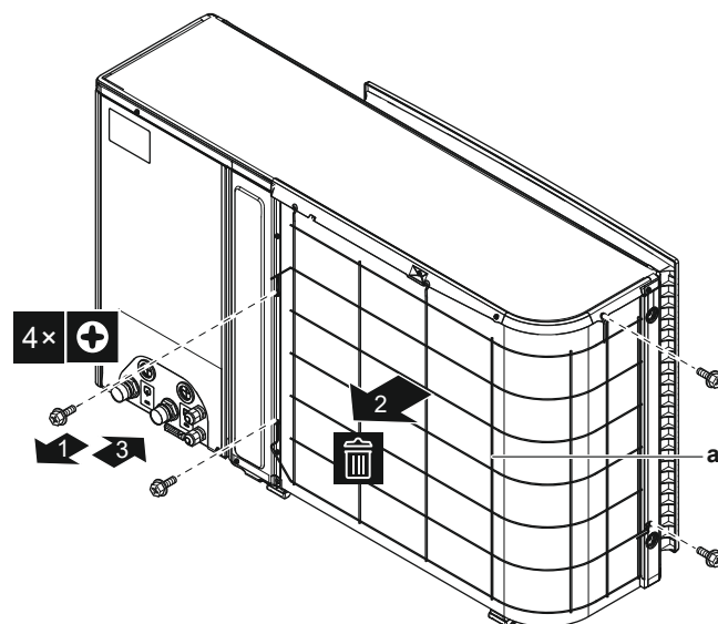
a Indsugningsgitter
