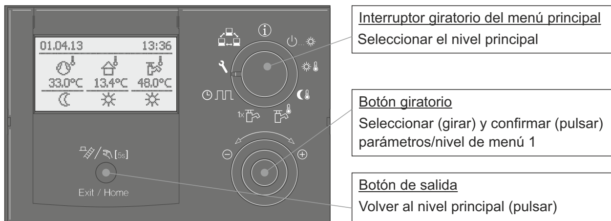
Figura 2-1 Regulador - Unidad de control
