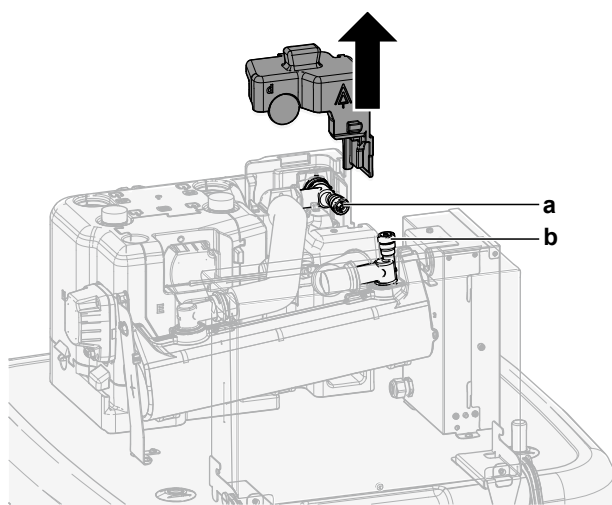
a, b Válvula de salida de ventilación manual
