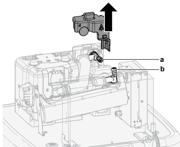
a, b Βάνα χειροκίνητου εξαρτισμού
