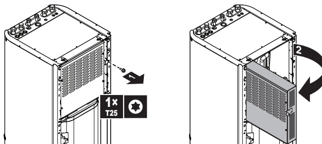
6 Περιστρέψτε τον ηλεκτρικό πίνακα.
