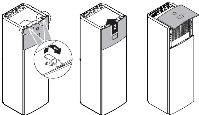
3 Αφαιρέστε την μπροστινή πλάκα.
