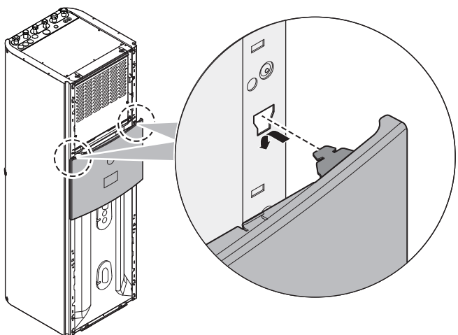
5 Αφαιρέστε το κάλυμμα του ηλεκτρικού πίνακα.
