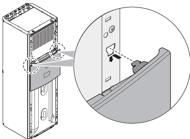
5 Свалете капака на превключвателната кутия.
