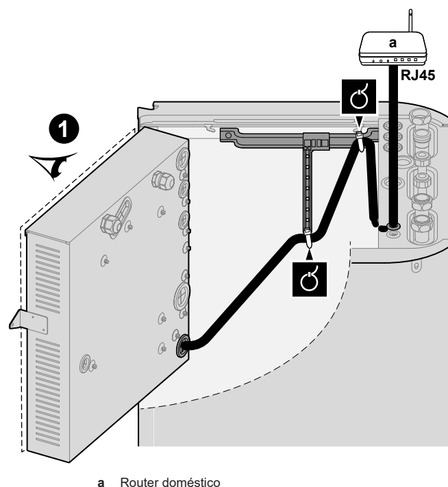
a Router doméstico
