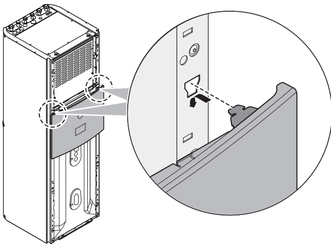
5 Fjern bryterboksdekselet.
