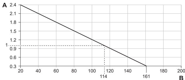
A Предварително налягане (bar) B Максимален обем на водата (l)
