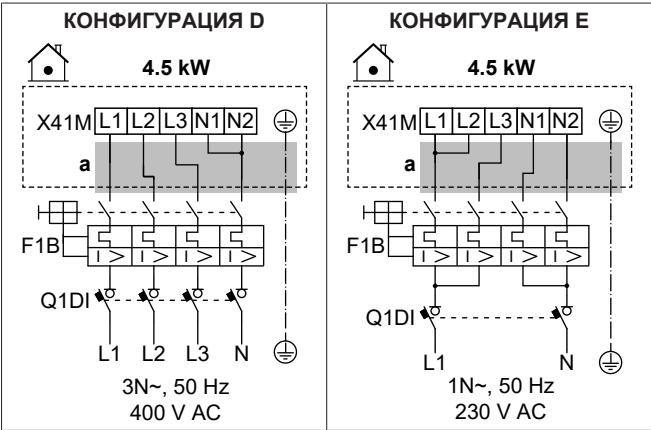
Възможни конфигурации при модели 4V (4,5 kW многостепенен резервен нагревател)
