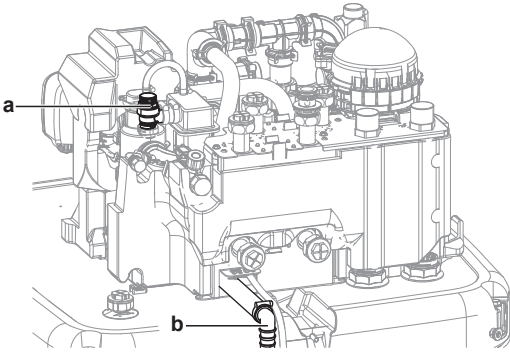
a Basınç boşaltma vanası b Basınç tahliye valfi bağlantısı
