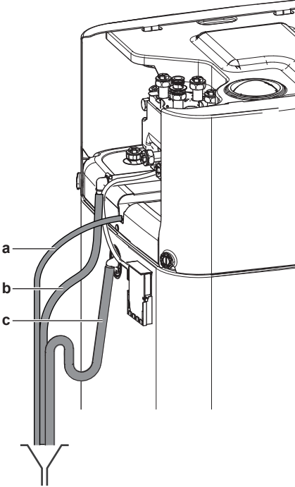
a Drenaj tavası hortumu (aksesuar olarak teslim edilir) b Drenaj hortumu basınç tahliye valfi (sahada temin edilir) c Drenaj hortumu deposu (sahada temin edilir)
