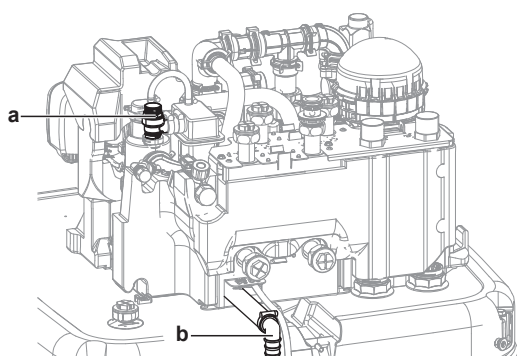
a Overdrukveiligheidsklep b Aansluiting drukveiligheidsklep
