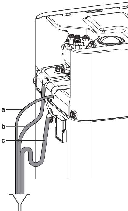
a Crijevo pitice za pražnjenje kondenzata (isporučuje se kao pribor) b Crijevo za pražnjenje ventila za ograničenje temperature i tlaka (lokalna nabava) c Spremnik crijeva za pražnjenje (lokalna nabava)
