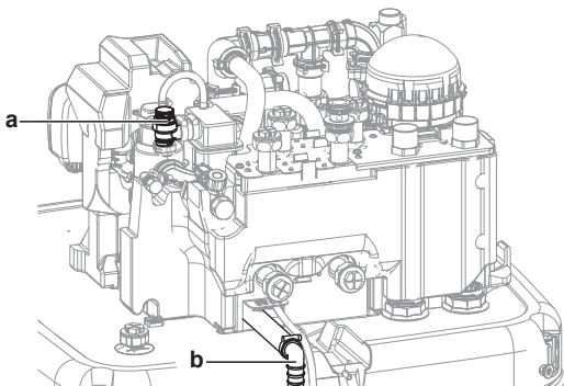
a Ventil za ograničenje tlaka b Priključak ventila za ograničenje tlaka
