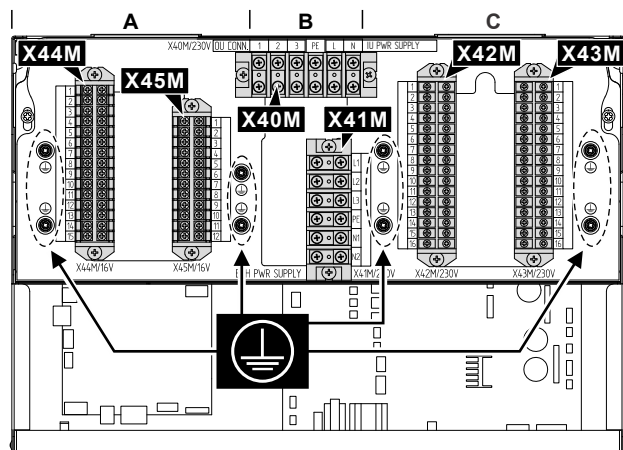
Terminalblokke (SWB1)
