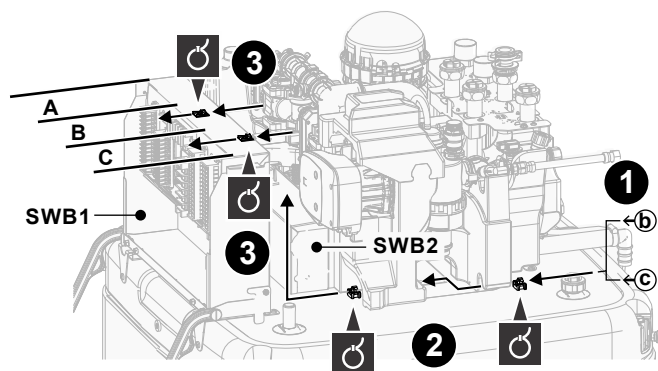
Terminalblokke (SWB1)
