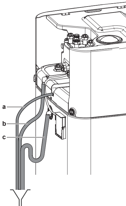
a Afløbsbakke (leveres som tilbehør) b Overtryksventil for afløbsslange (medfølger ikke) c Afløbsslangetank (medfølger ikke)
