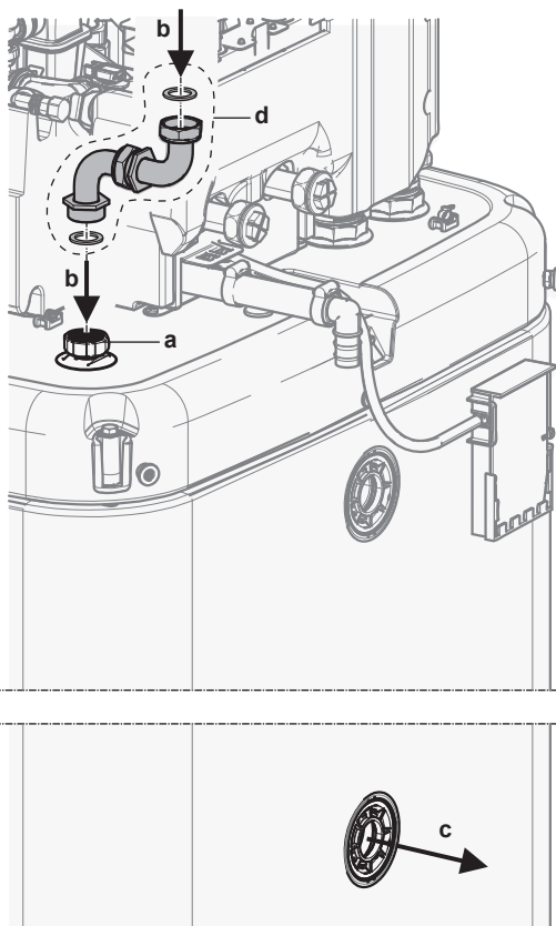
a Złącze drainback
