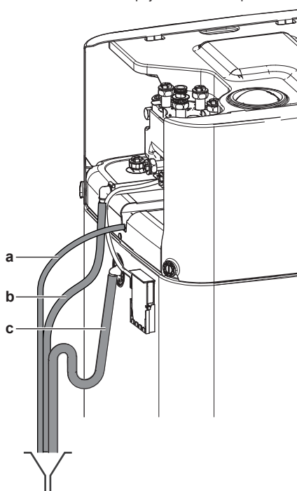
a Hadica odtokovej vane (dodáva sa ako príslušenstvo) b Tlakový poistný ventil odtokovej hadice (napájanie v teréne) c Nádrž vypúšťacej hadice (napájanie v teréne)
