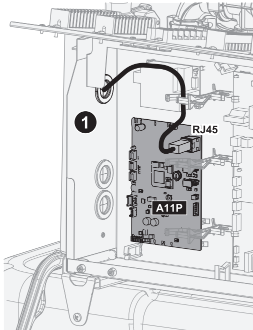
Verlegung bei 90°-Verbindung
