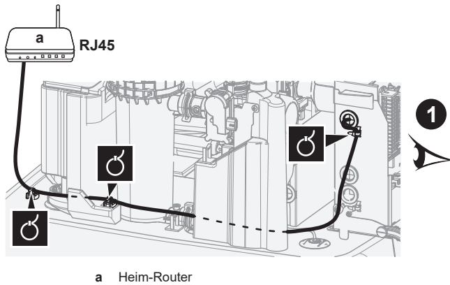
Verlegung bei geradem Stecker
