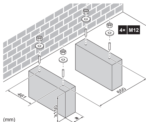
a Attenzione a non coprire il foro di scarico della piastra sul fondo dell'unità.
