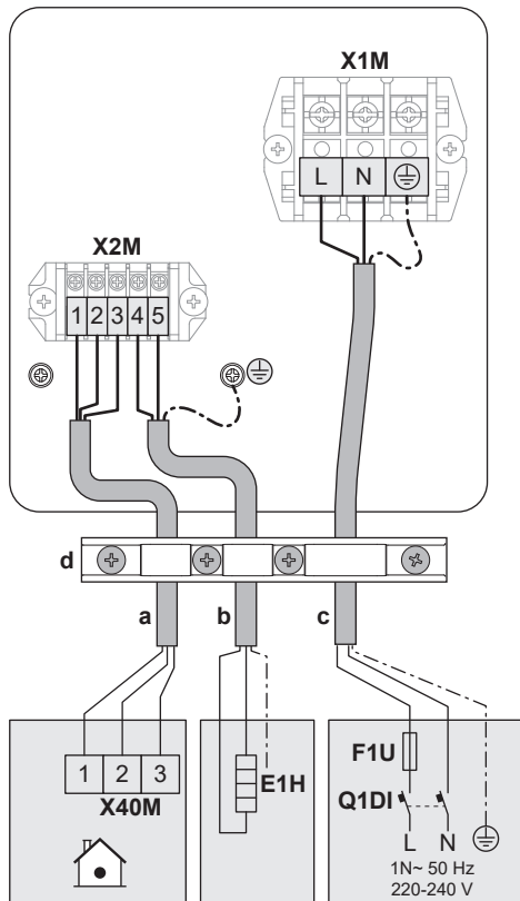
Kabelübersicht: V3-Modelle (1N~)
