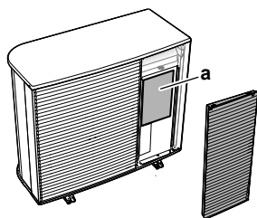
а Электрическая схема
