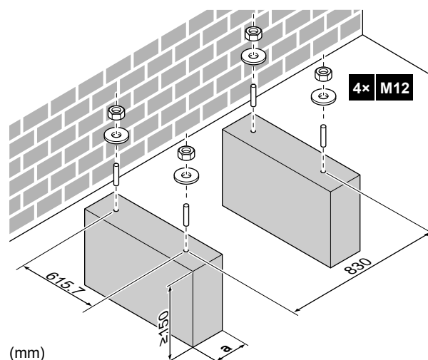
a Nesmíte zakrýt vypouštěcí otvor ve spodní desce jednotky.
