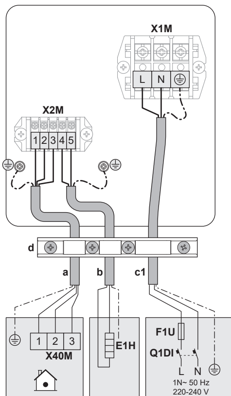
Схема на кабелите: модели V3 (1N~)
