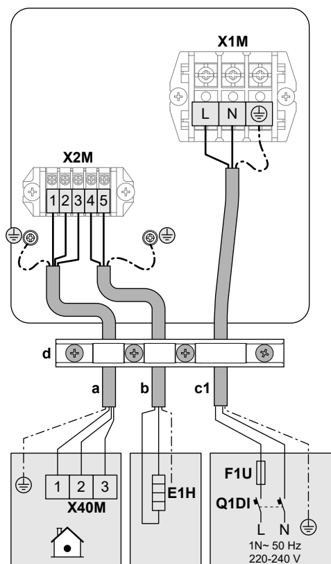
Схема на кабелите: модели W1 (3N~)
