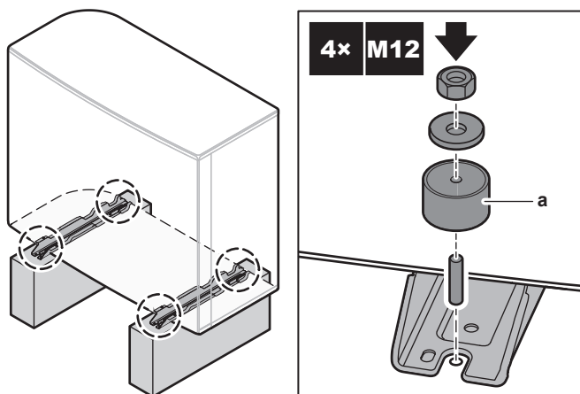
a Противовибрационная резина (приобретается на месте)
