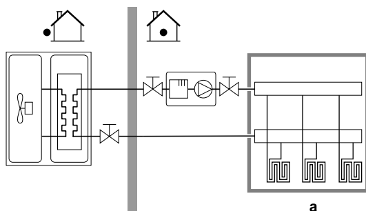
a LWT-hovedzone
