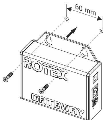
Afbeelding 2: Wandmontage
