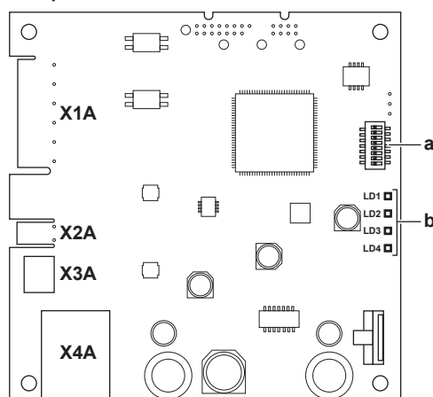
X1A~X4A Connecteurs a Microcommutateur b Diodes électroluminescentes d'état
