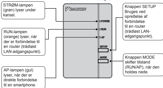
Trådløs LAN-adapter
