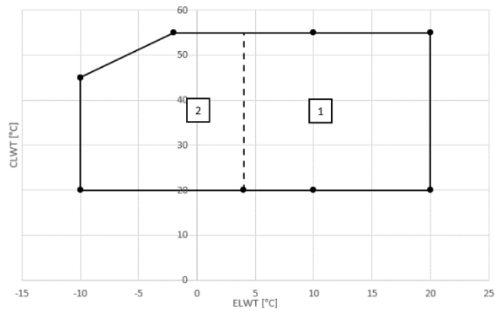
Afbeelding 4 - Werkingslimieten EWWQ049-064
