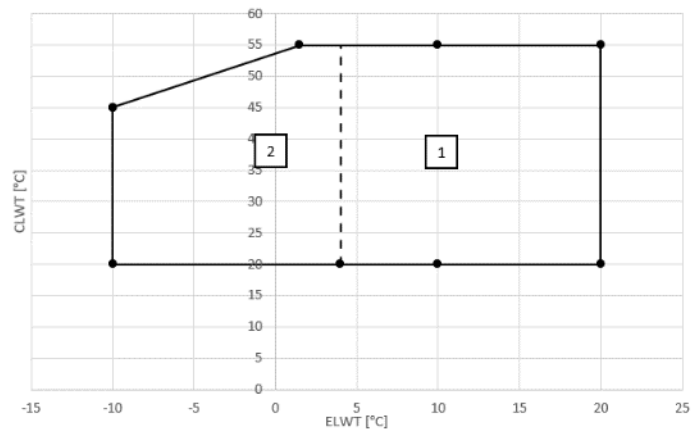
Afbeelding 3- Werkingslimieten op EWWQ014-033
