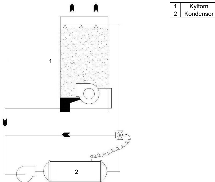
Figur 12 - Kondensorns kontrollschema med kyltorn
