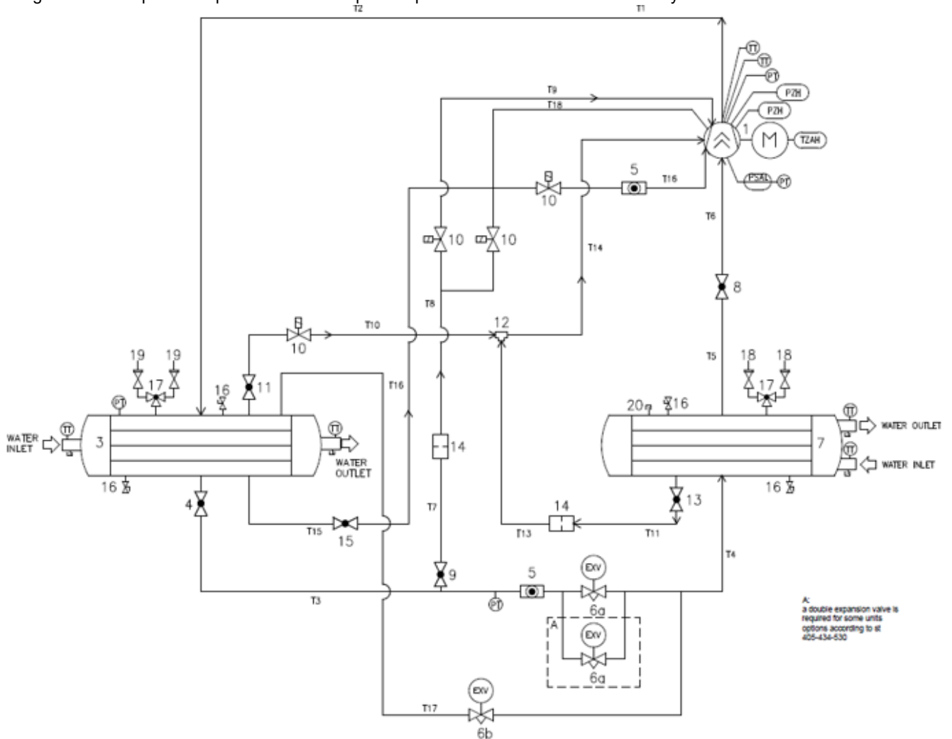
Figura14 - P&ID Opción.251
