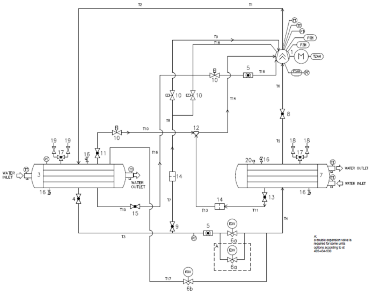
Abbildung14 - P&ID Option 251
