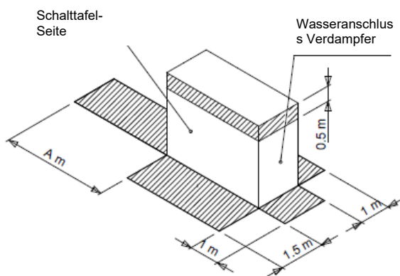
Abbildung4 - Positionierung des Geräts
