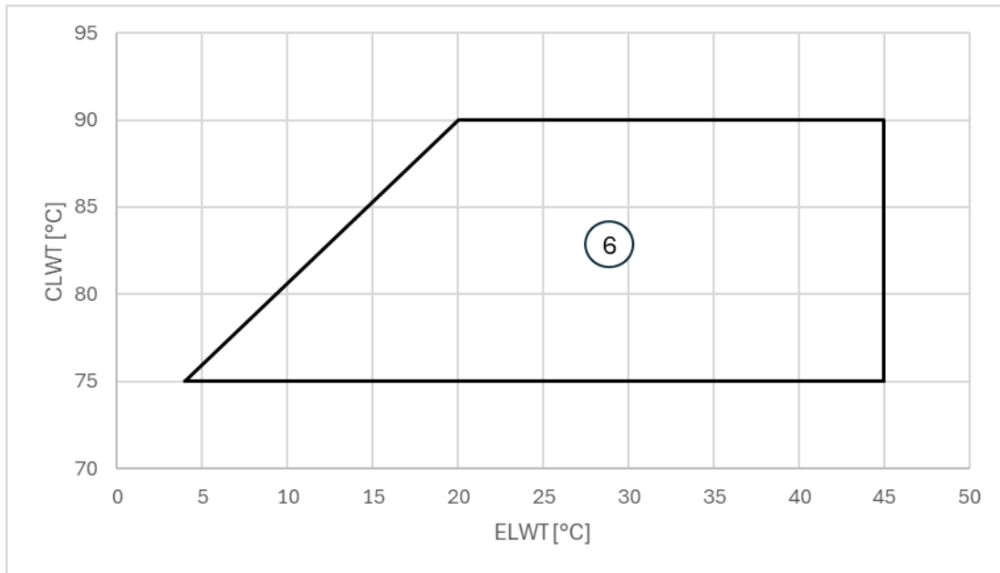
Abbildung9 - EWWH_VZ_XS/PS Option 251
