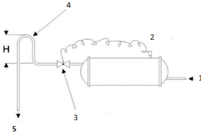
Abbildung13 - Kondensatorkontrollschema mit Brunnenwasser
