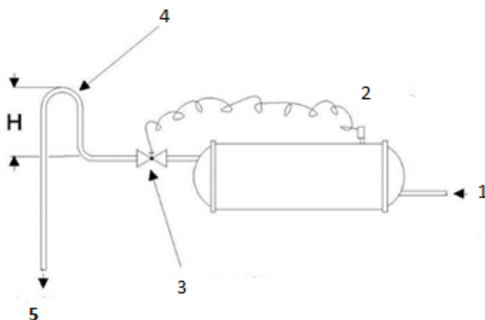
Figur 13 - Kondensorns kontrollschem med behållarvatten
